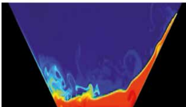
Modelo numérico complejo calculado para ajustarse al tsunami local generado por un deslizamiento de tierras en bahía Lituya (Alaska) en 1958, que provocó el mayor runup jamás registrado (525 m). Este modelo complejo ajusta de forma precisa el detalle de los vórtices de segundo orden y los efectos de las salpicaduras demostrados por los experimentos de laboratorio. Cortesía de Galen Gisler (Laboratorio Nacional de Los Álamos).
