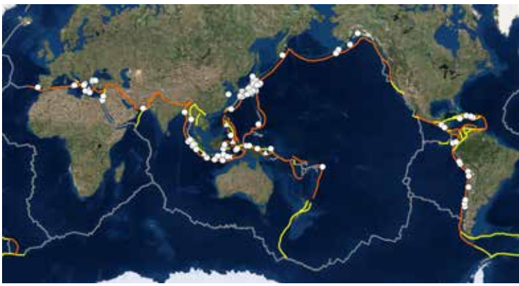
Localización de las fuentes de tsunamis en el mundo. Los tsunamis pueden ocurrir en cualquier momento y en cualquier lugar de convergencia o subducción activa de las placas tectónicas (líneas naranjas). El riesgo de tsunami existe en todos los océanos y cuencas, pero ocurren con más frecuencia en el océano Pacífico. Se muestran tsunamis históricos que causaron más de 100 muertes. La mayoría fueron generados por terremotos (círculo), y unos pocos por erupciones volcánicas (triángulo). Las zonas de subducción se muestran en naranja, el relieve dorsal oceánico activo en gris y las fallas transformantes en amarillo. Fuente: NCEI/Sistema Mundial de Datos Geofísicos, LDG-DASE, ITIC.
